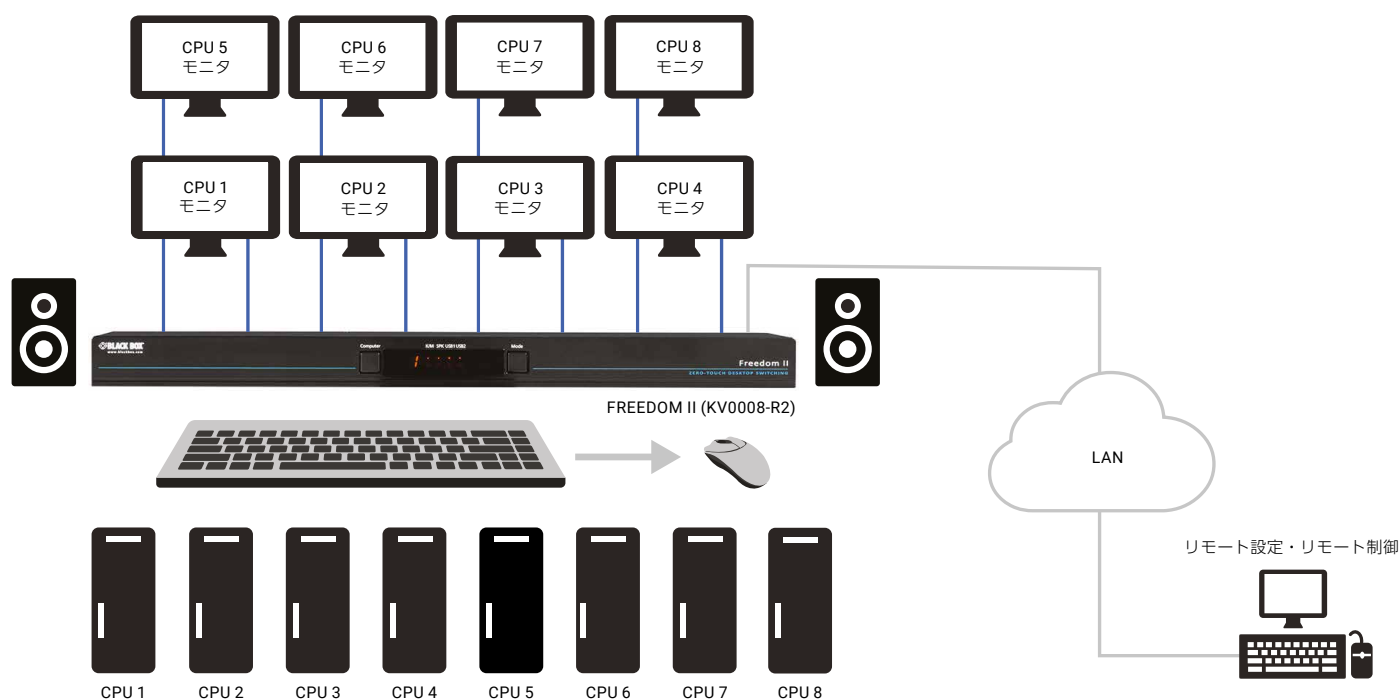
8ポート構成 Freedom II
