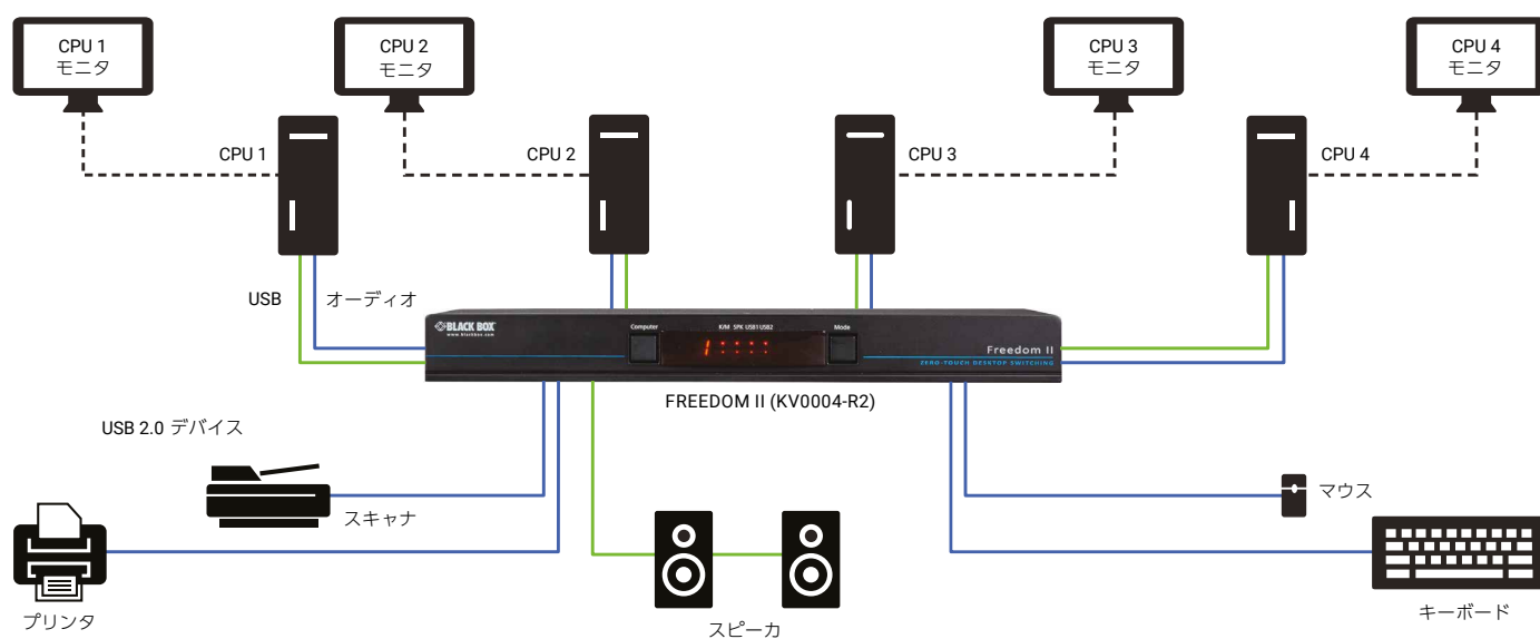
4ポート構成のFreedom II (USB 2.デバイス)
